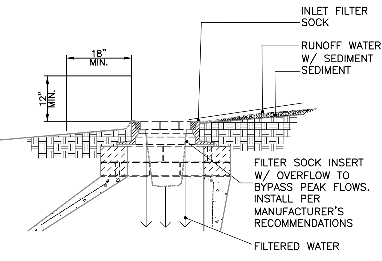
2 INLET PROTECTION DETAIL SCALE: N.T.S.
