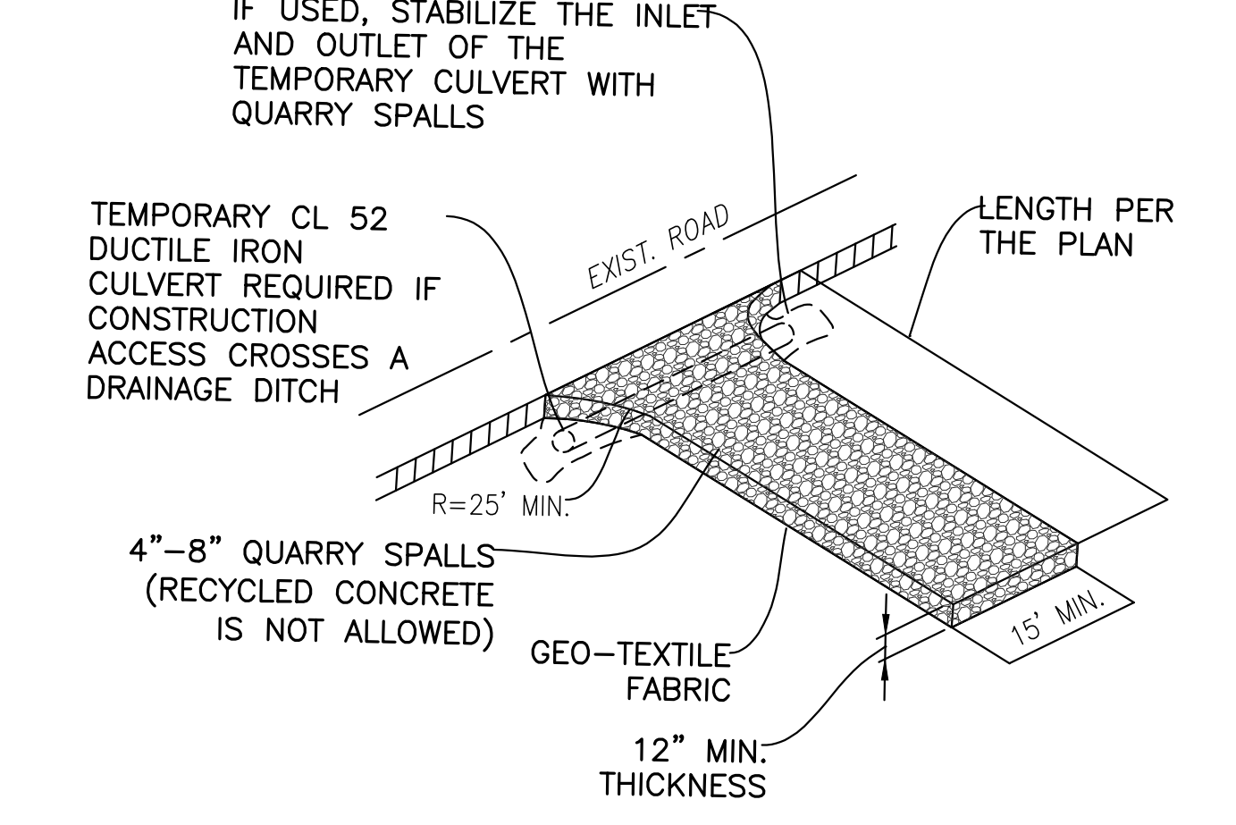
4 STABILIZED CONSTRUCTION ACCESS SCALE: N.T.S.
