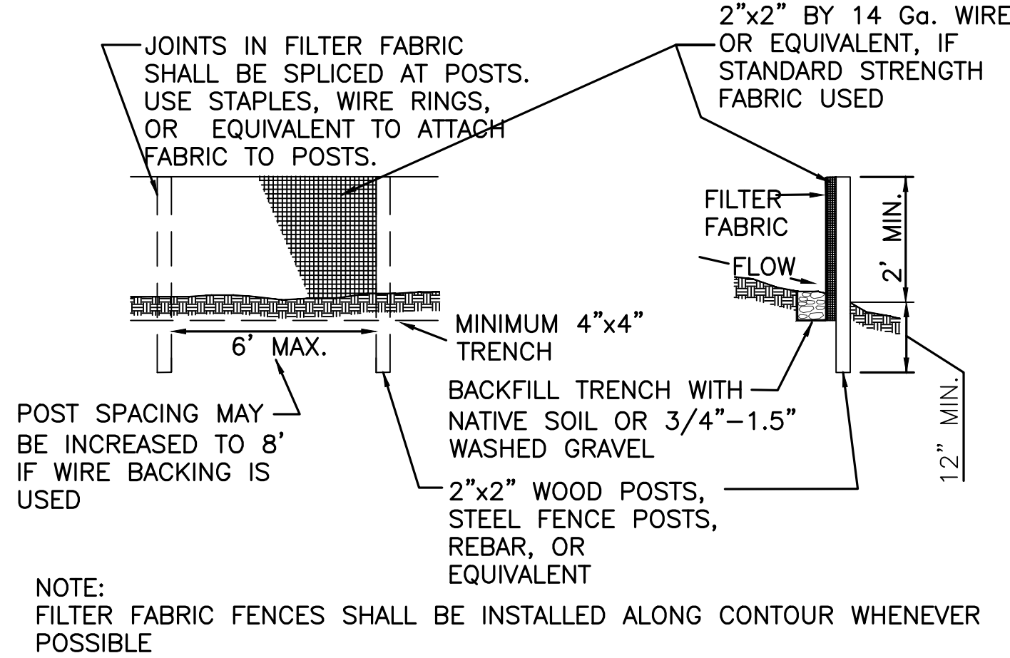
3 SILT FENCE DETAIL SCALE: N.T.S.
